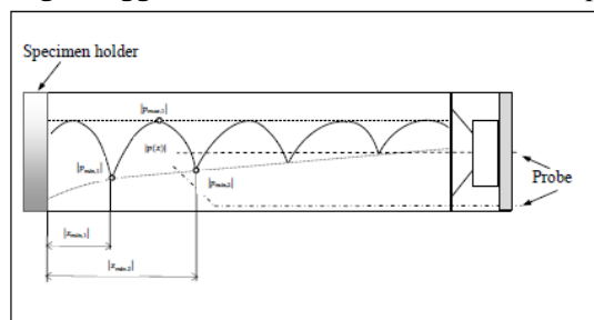
Gambar 2.3. Pandangan skematis metode rasio gelombang tegak.
